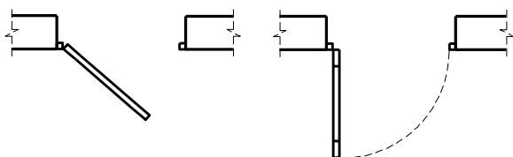
a) Cửa đi bản lề đứng không có ngưỡng cửa
