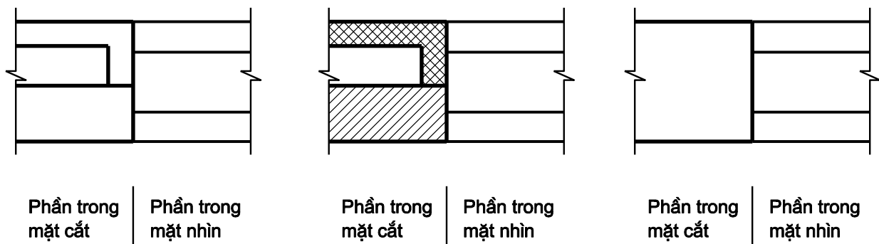
Hình 1 - Ví dụ về các đường bao ngoài của các phần trong mặt cắt và mặt nhìn
