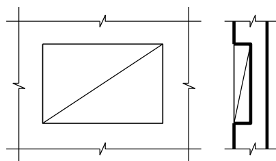
Hình 10 - Hốc tường
