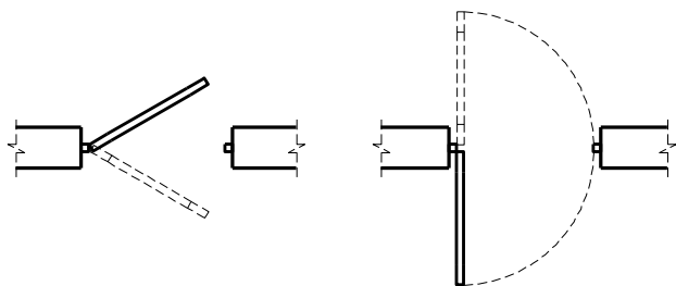
c) Cửa đi mở hai phía
