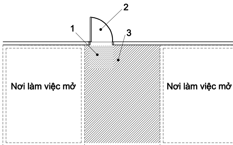
Hình 11 - Phòng kỹ thuật được bố trí lùi sau diện tích giao thông
