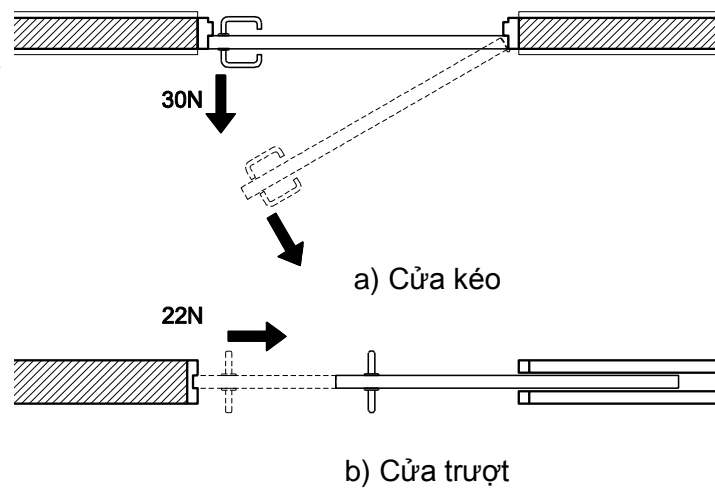
Hình 14 - Lực đóng mở cửa
