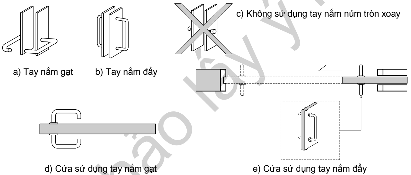
Hình 13 - Chi tiết tay nắm cửa
