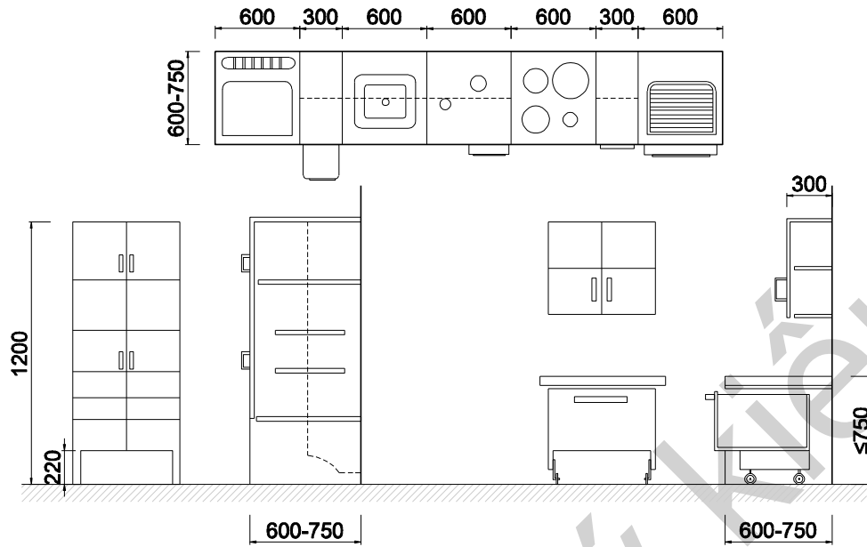
a) Kích thước bàn bếp, tủ bếp
