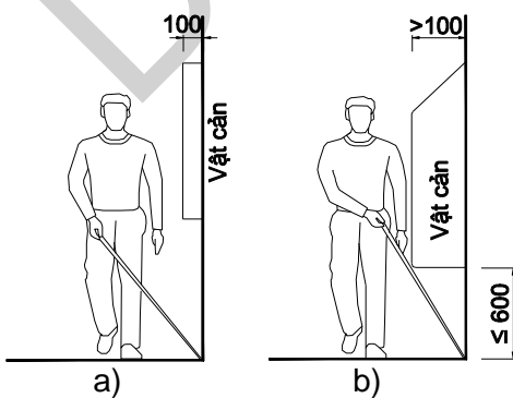
Hình 18 - Quy định kích thước vật gắn trên tường
