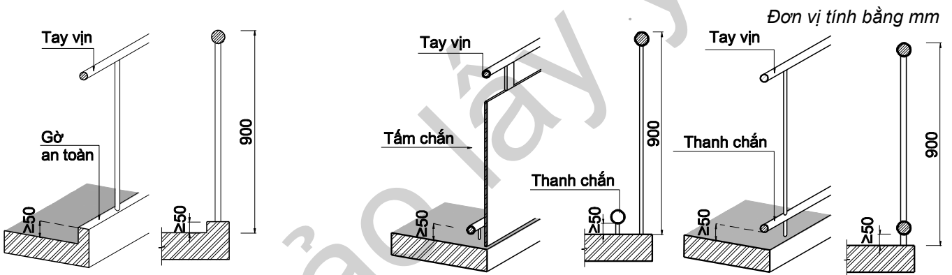
a) Gờ an toàn chân lan can
