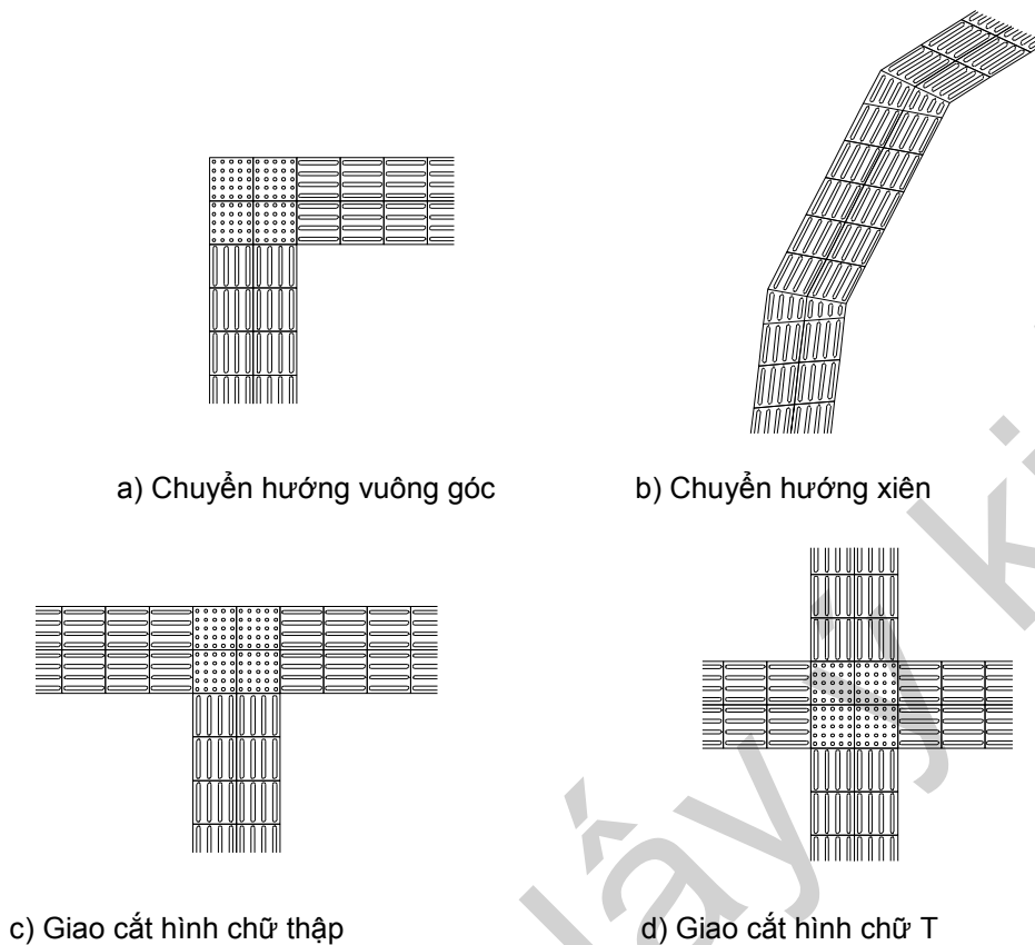
Hình 49 - Bố trí tấm lát dẫn hướng tại vị trí có sự chuyển hướng
