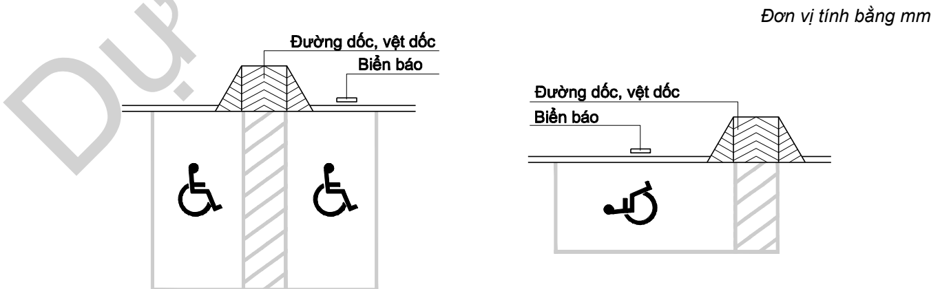
Hình 1 - Chỗ để xe ô tô
